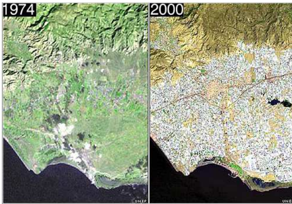
Vista satelital del litoral almeriense entre 1974 y 2000
